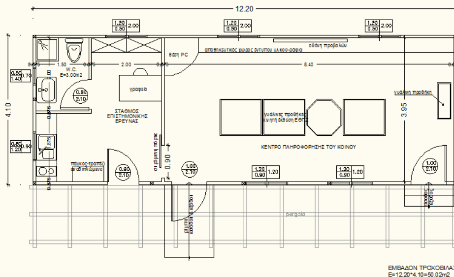
ΕΝΔΕΙΚΤΙΚΟ ΣΧΕΔΙΟ ΤΡΟΧΟΒΙΛΑΣ
