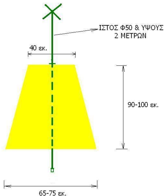
ΣΚΑΡΙΦΗΜΑ ΚΩΝΙΚΟΥ ΣΗΜΑΝΤΗΡΑ
