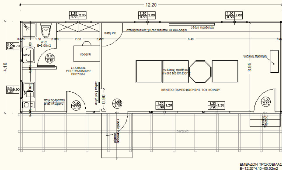
ΕΝΔΕΙΚΤΙΚΟ ΣΧΕΔΙΟ ΤΡΟΧΟΒΙΛΑΣ
