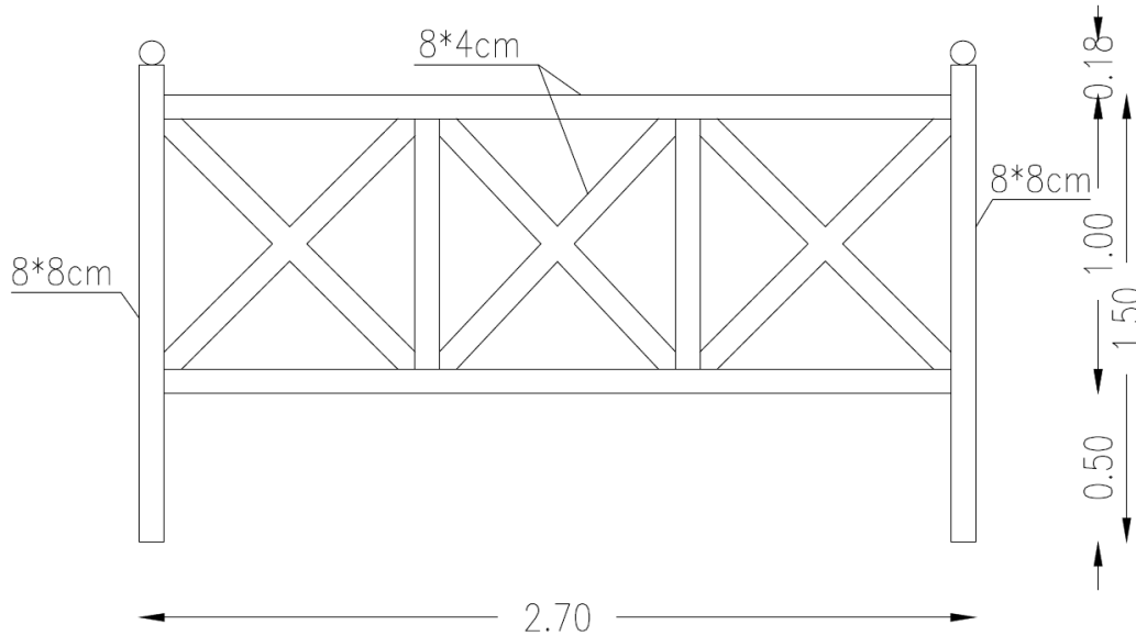
Σχέδιο 1. Μεταλλικές Μπάρες
